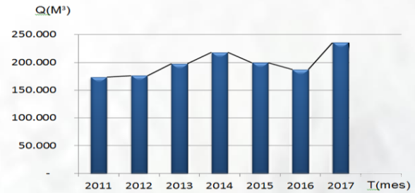
Figura 3. Producción de agua potable en Roldanillo
